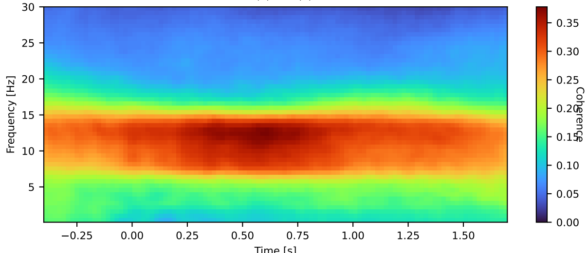
8B (1) - 8B (2)
